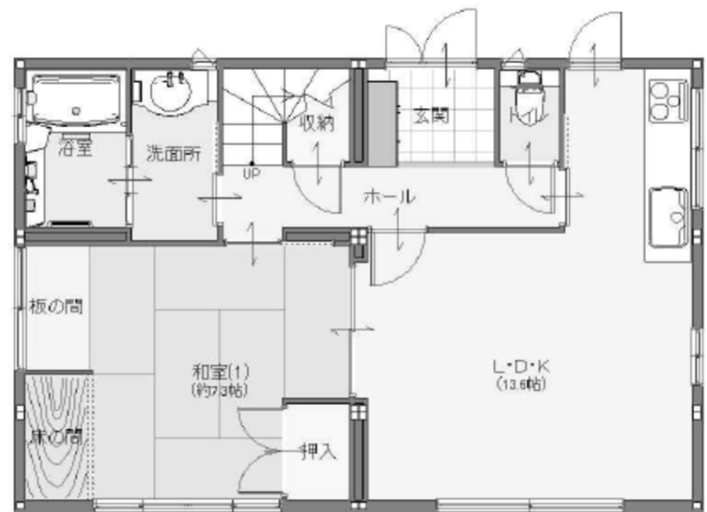
1階
