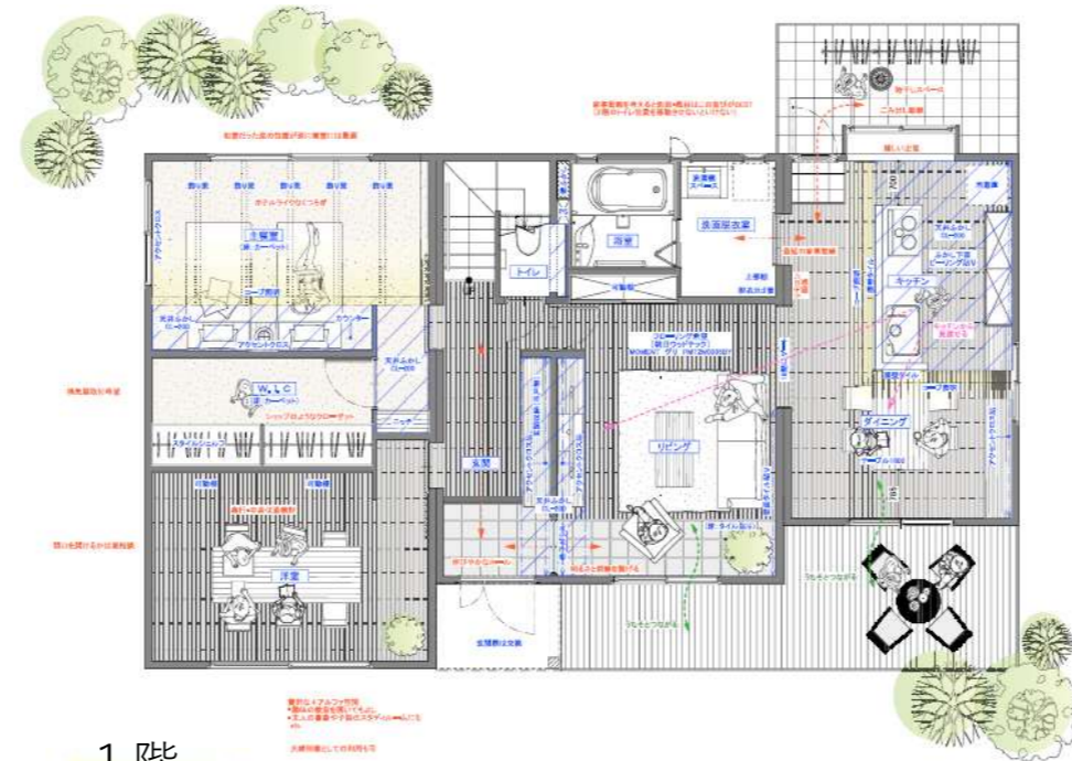
1階
